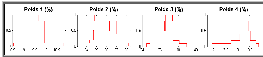
Figure 5 : Résultats de l'extension floue de RLMC-étendu sur le problème défini en figure 4
