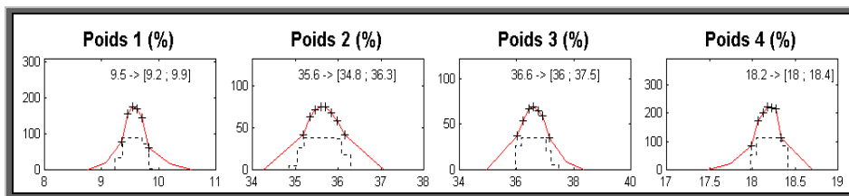
Figure 6 : Résultats d'une simulation de Monte Carlo à partir de la méthode RLMC-étendu sur le problème défini en figure 4
