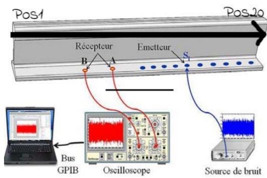
Fig1: Dispositif expérimental [3]
