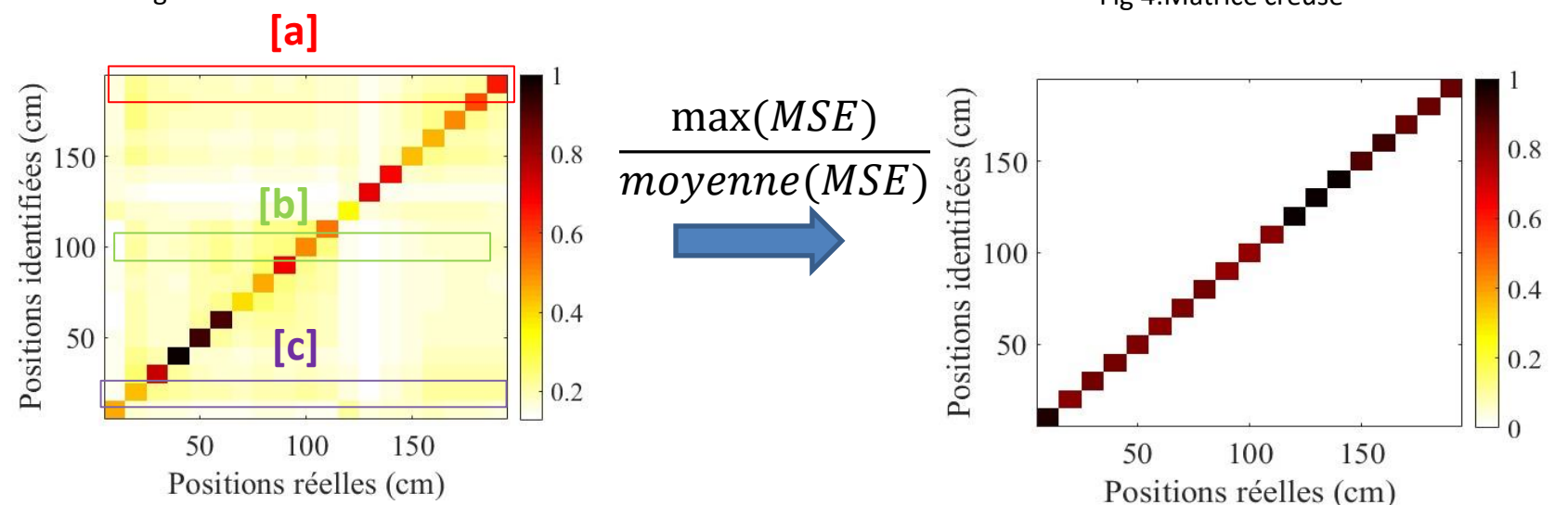
Fig 3: Matrice cohérente.
