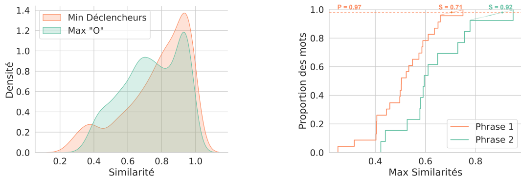
(a) Similarités : min déclencheurs VS max « O »
