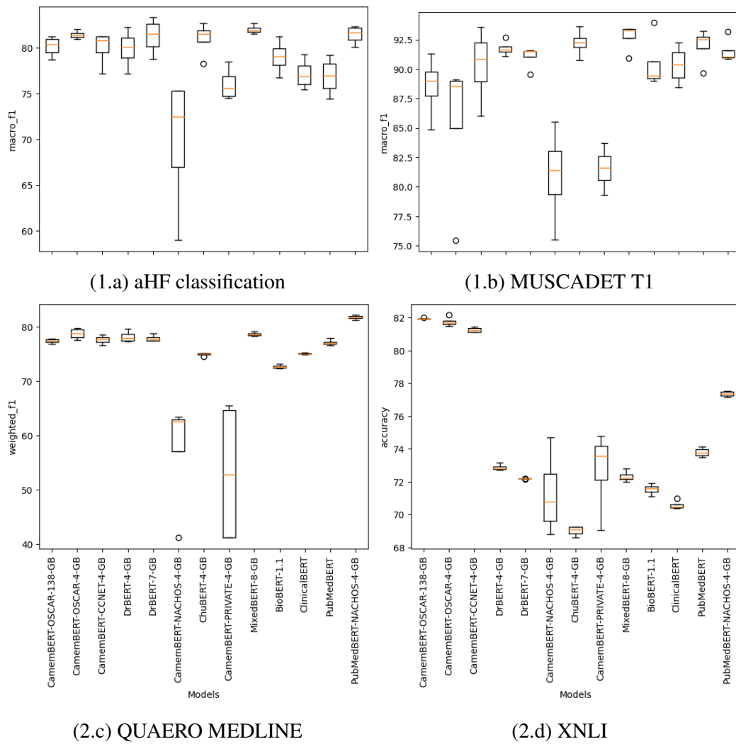
FIGURE 2 – Boîte à moustaches pour chaque modèle.
