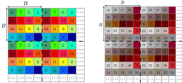
FIGURE 1 – MSFAs utilisés : IMEC VIS 4 \times 4 ( \lambda^b \in \{469 \text{ nm}, \dots, 633 \text{ nm}\} , b \in \llbracket 0, 15 \rrbracket ) (gauche) et NIR 5 \times 5 ( \lambda^b \in \{678 \text{ nm}, \dots, 960 \text{ nm}\} , b \in \llbracket 0, 24 \rrbracket ) (droite).
