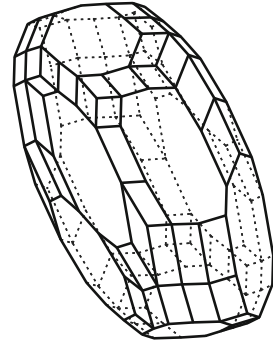
(D) Another generic 3rd higher 6-permutahedron.
