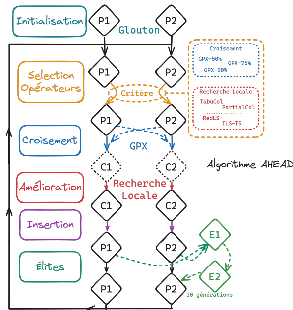
FIG. 1 – Architecture générale de l'algorithme AHEAD.
