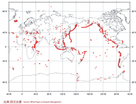
FIG. 7 : Cartes de répartition des volcans dans le monde et des tremblements de terre à l'origine de tsunamis sur la côte Est du Japon (source Gouvernement, 2022)
