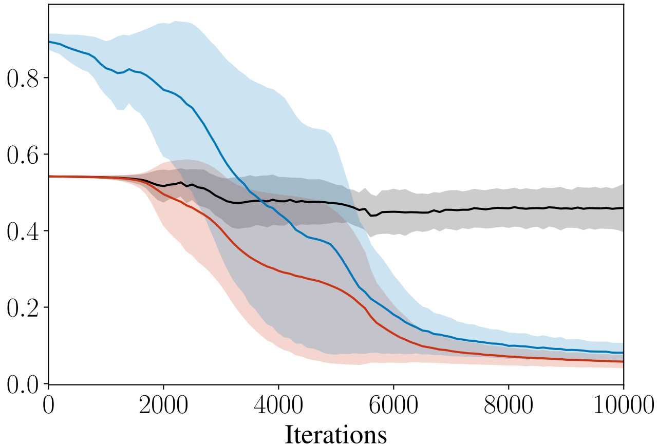
MNIST
