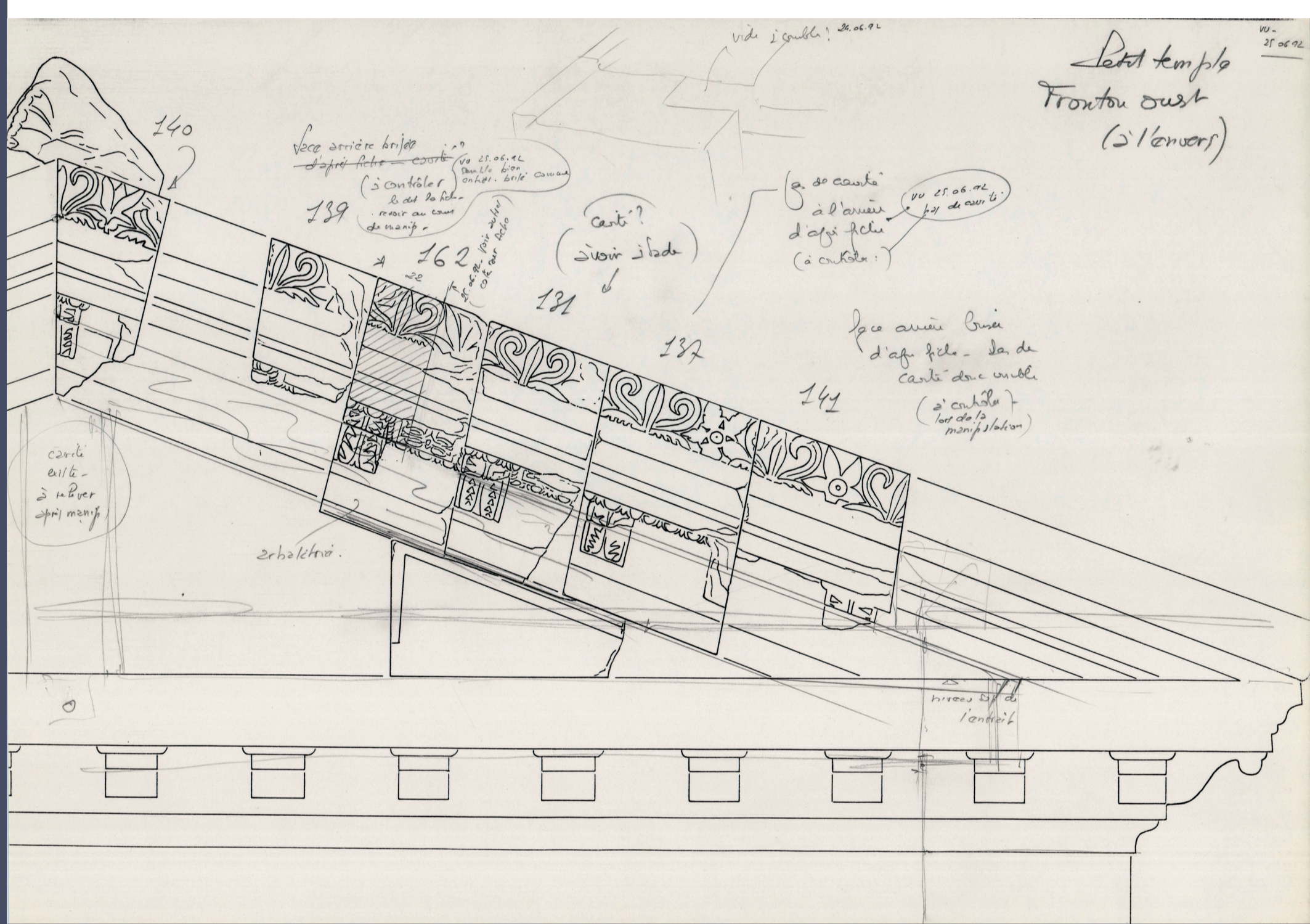
Fig. 2 : Dessin de Pierre Varène représentant l'attribution et le positionnement de blocs de corniche rampante. Restitution d'une moitié du fronton du petit temple de Glanum réalisé en 1992 dans le cadre de l'opération de reconstruction partielle du monument. Cet exemple montre le nécessaire travail de recontextualisation pour rendre ce document intelligible à des non-spécialistes.
