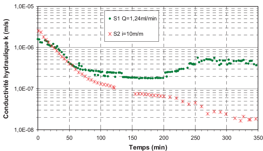
Figure 6. Conductivité hydraulique en fonction du temps
