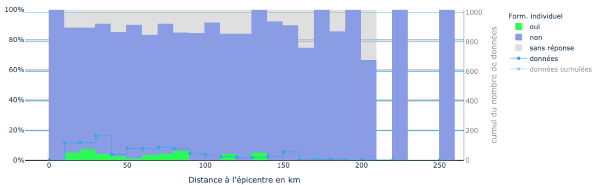
Figure 2.14 - Sortie des bâtiments en courant par les témoins. (formulaire individuels).
