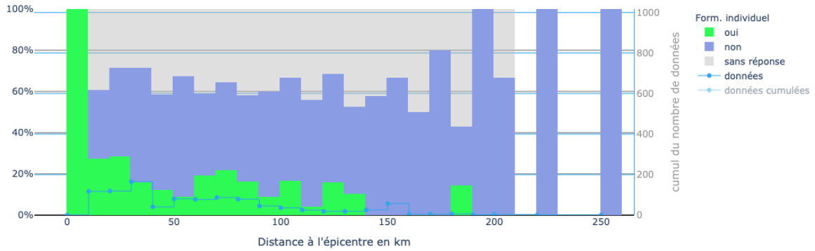
Figure 2.12 - Bruits ressemblant à un coup de tonnerre proche et fort par distance épacentrale. (formulaire individuels)
