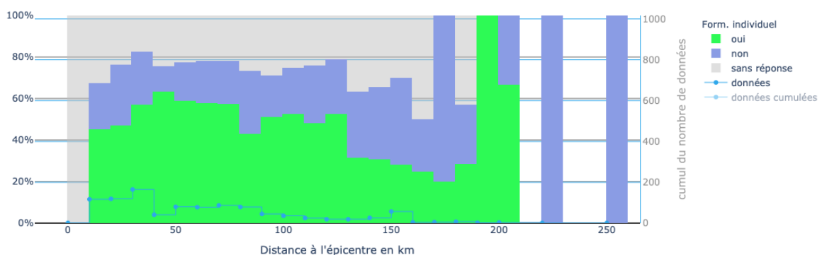
Figure 2.11 - Bruits ressemblant à un grondement faible et lointain par distance épicentrale. (formulaire individuels)
