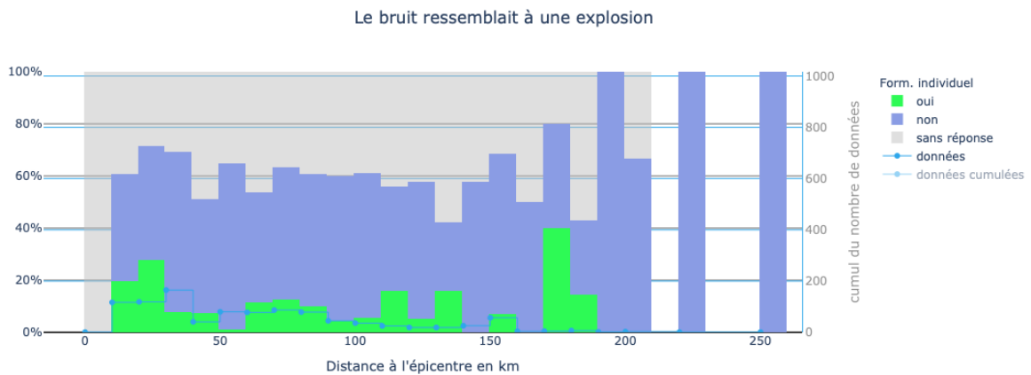
Figure 2.13 - Bruits ressemblant à explosion par distance épacentrale. (formulaire individuels)
