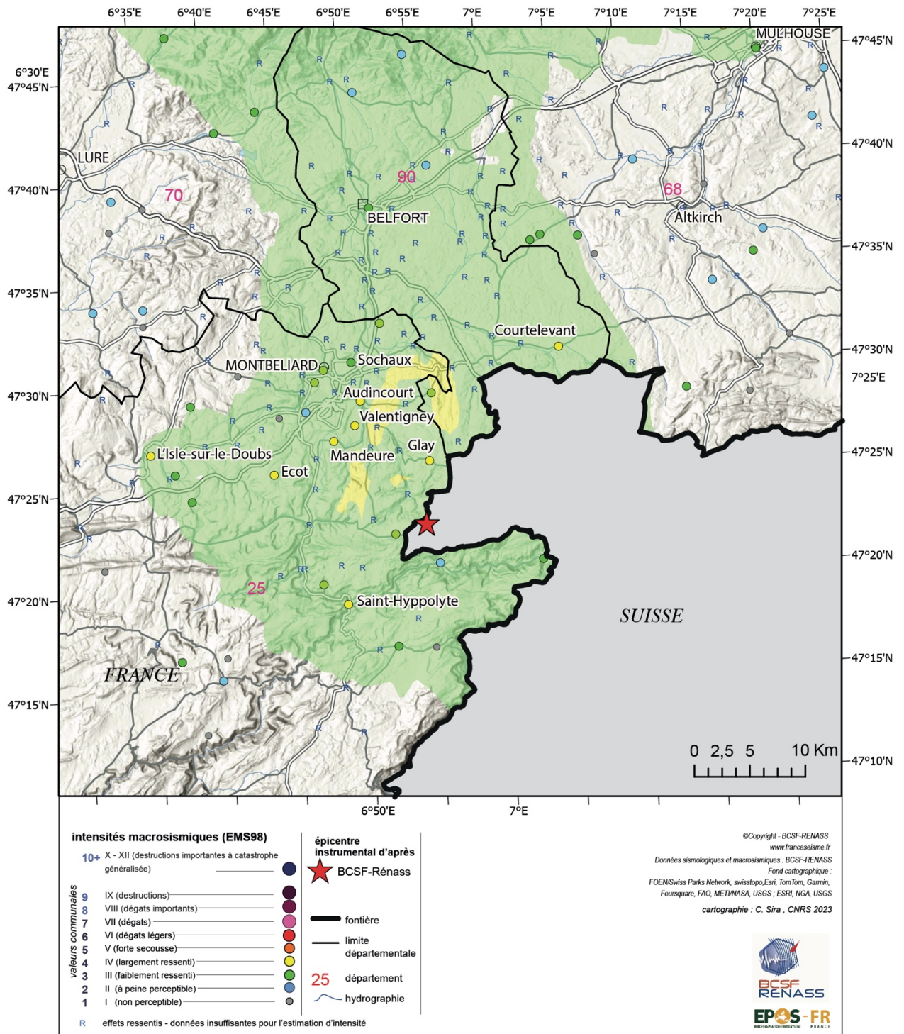
Figure 2.1 – Carte d'intensités macrosismiques de la zone épacentrale.
