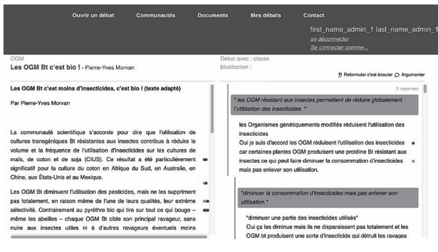
Figure 1 Présentation de l'interface de la plateforme
