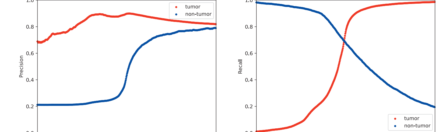
Figure 10 : Précision (a) et rappel (b) en fonction du seuil choisi en ACP.
