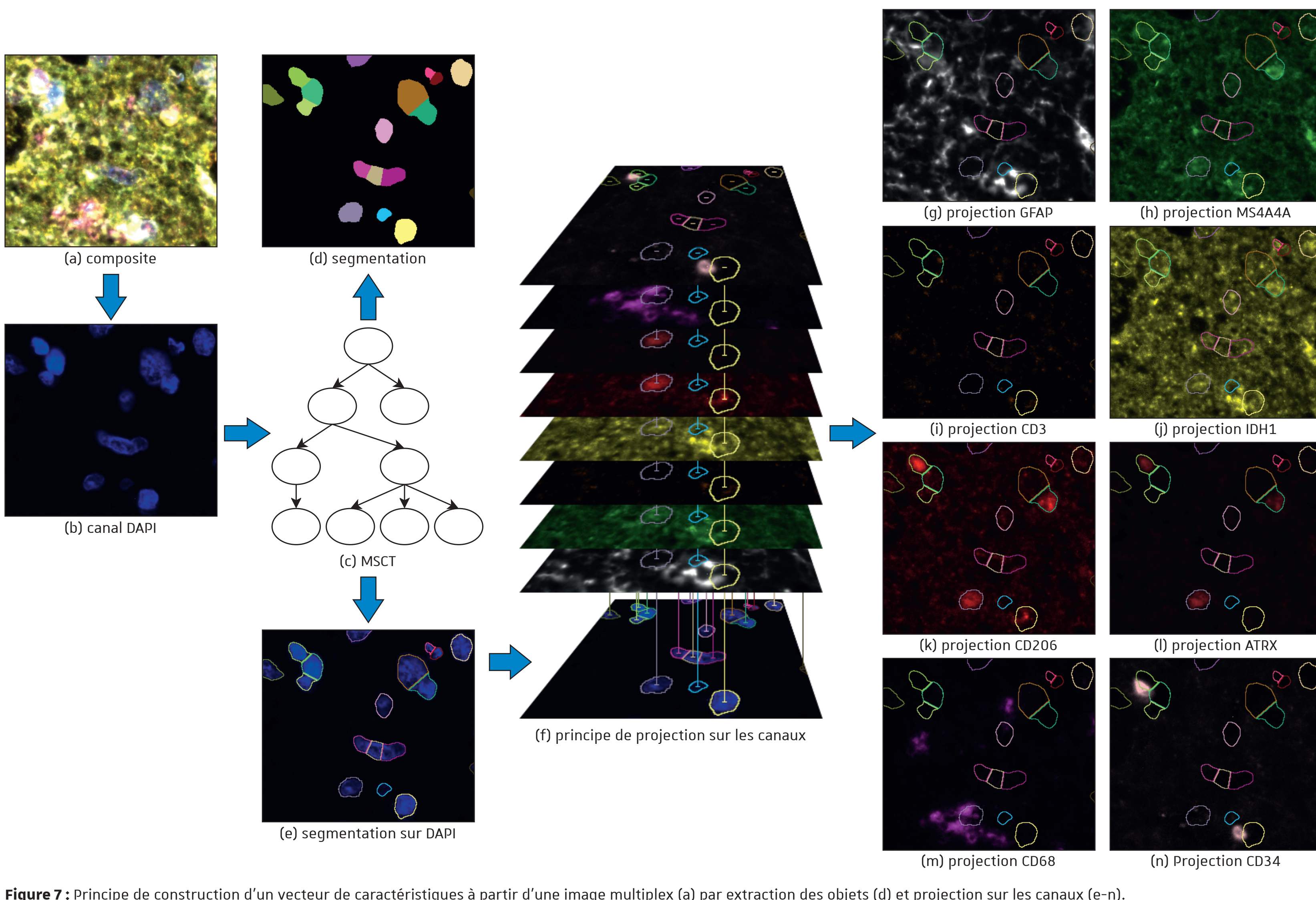
Figure 7 : Principe de construction d'un vecteur de caractéristiques à partir d'une image multiplex (a) par extraction des objets (d) et projection sur les canaux (e-n).
