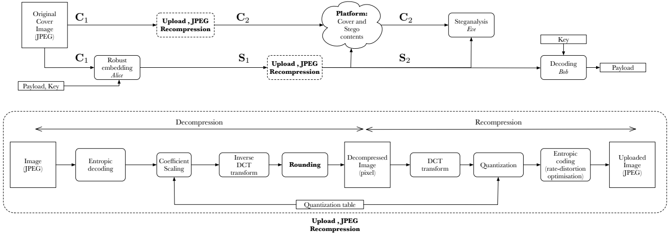
FIGURE 1 – Schéma considéré pour une stéganographie robuste après compression JPEG : le diagramme du haut représente l'ensemble de la chaîne de traitement et les différents acteurs (Alice, Bob et Eve). Le diagramme du bas décrit les différentes opérations impliquées dans le processus de téléversement sur la plateforme.
