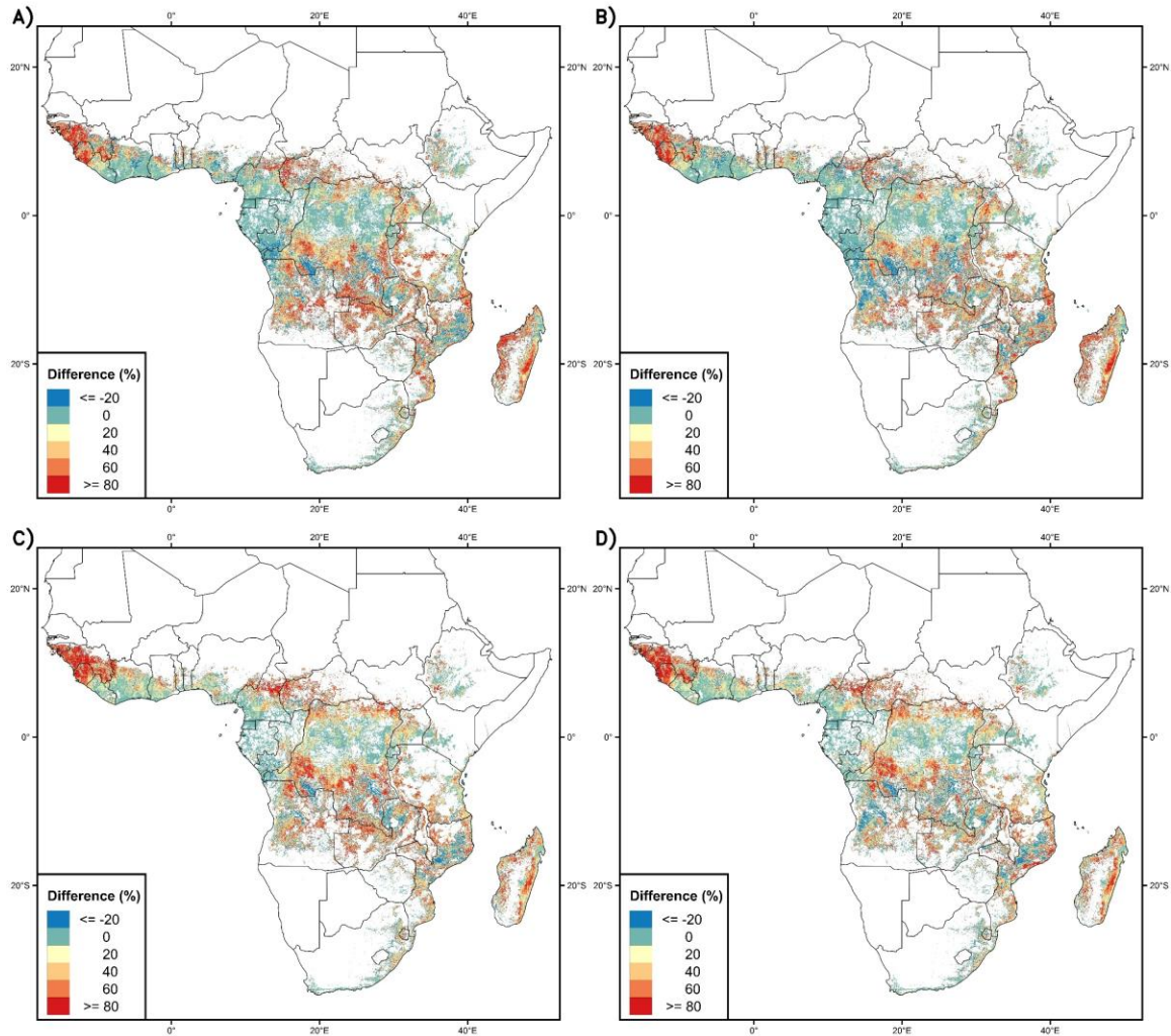
Fig. 5 | Differences of fire-related forest loss estimations: (A) FireCCISFD – MCD64A1 (2016); (B) FireCCISFD – FireCCI51 (2016); (C) FireCCISFD – MCD64A1 (2019); (D) FireCCISFD – FireCCI51 (2019)
