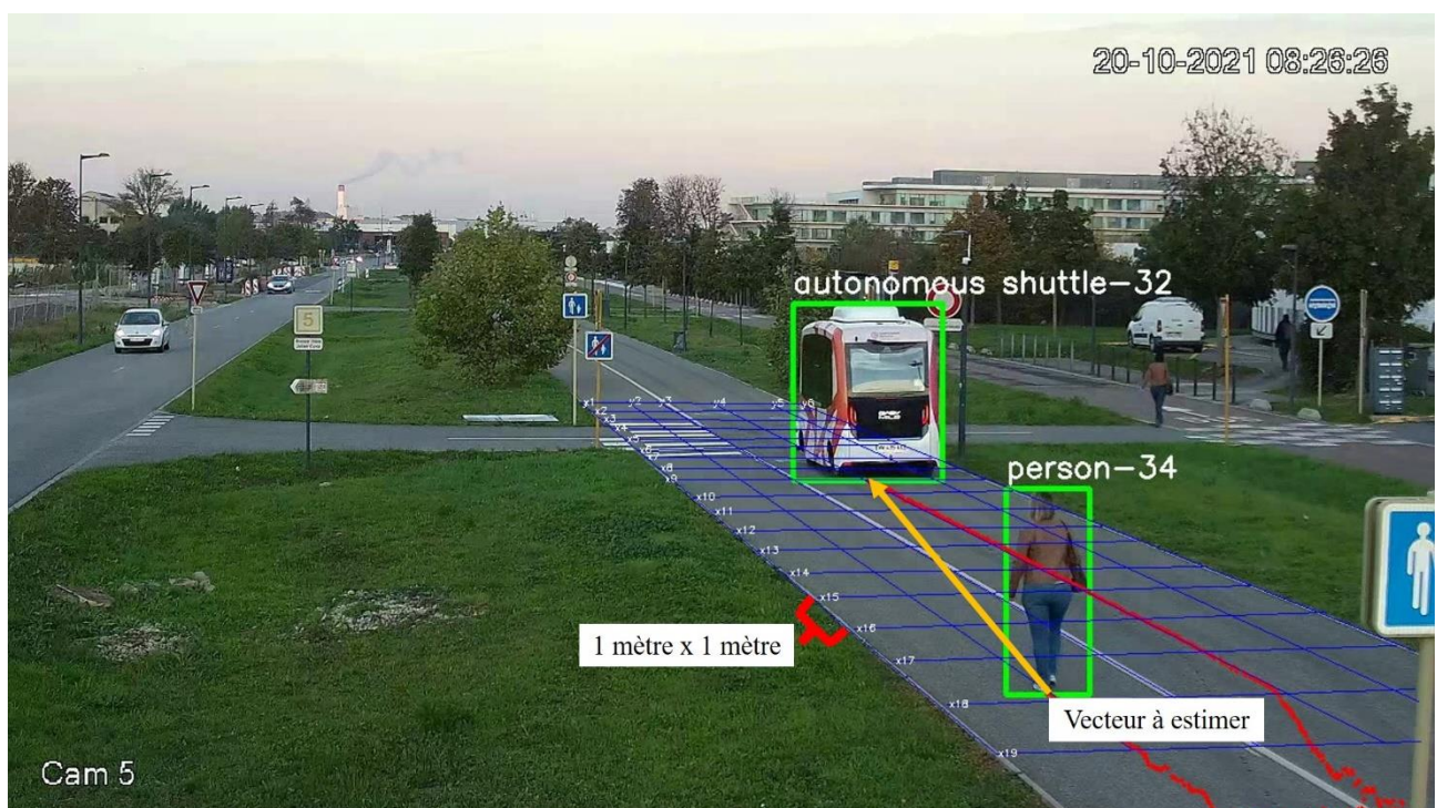
Figure 19. Grille avec des carrés de 1 mètre x 1 mètre utilisée pour estimer la distance entre les objets de la scène.
