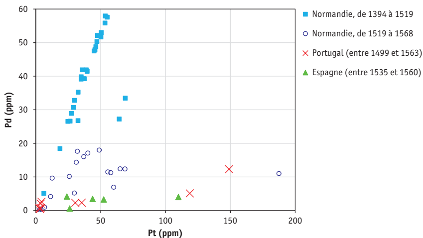
Figure 4 - Teneurs en palladium (Pd) en fonction de celles en platine (Pt) de monnaies d'or émises en Normandie entre 1394 et 1568 et au Portugal et en Espagne dans la 1 re moitié du XVI e siècle.
