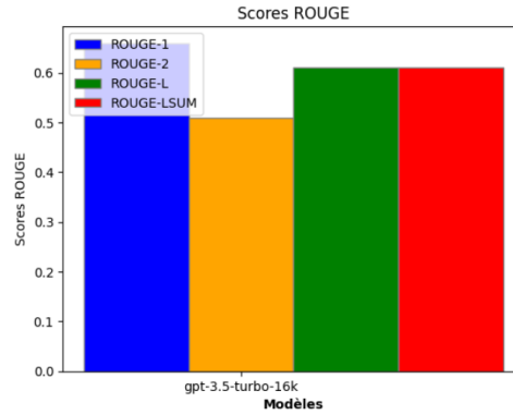
Fig. 15. ROUGE gpt-3.5-turbo-16k.
