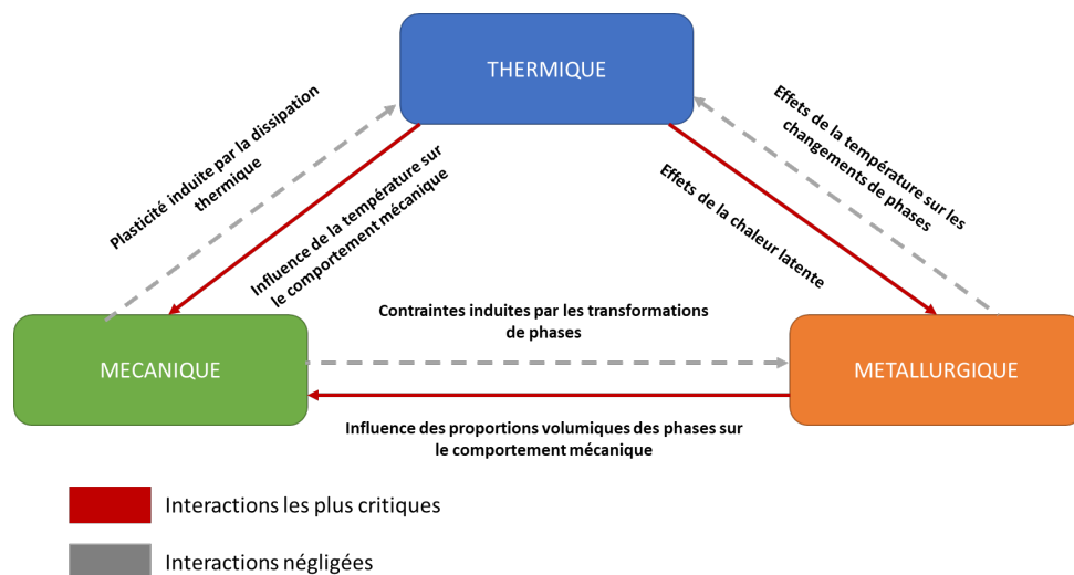
FIGURE 1 – Couplage en modélisant les effets thermiques, métallurgiques et mécaniques.
