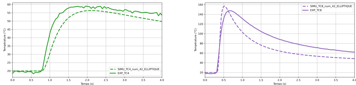
(a) Thermocouple en surface situé à 1.3 mm de hauteur au passage de la meule. (b) Thermocouple à 5 mm de profondeur situé à 1.3 mm de hauteur au passage de la meule.
