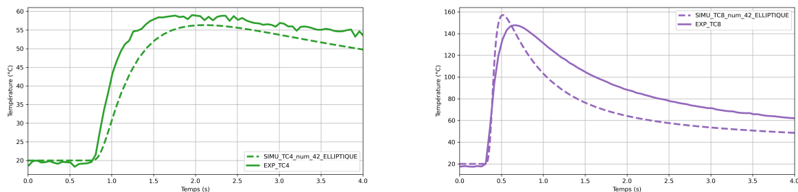
(a) Thermocouple en surface situé à 1.3 mm de hauteur au passage de la meule. (b) Thermocouple à 5 mm de profondeur situé à 1.3 mm de hauteur au passage de la meule.
