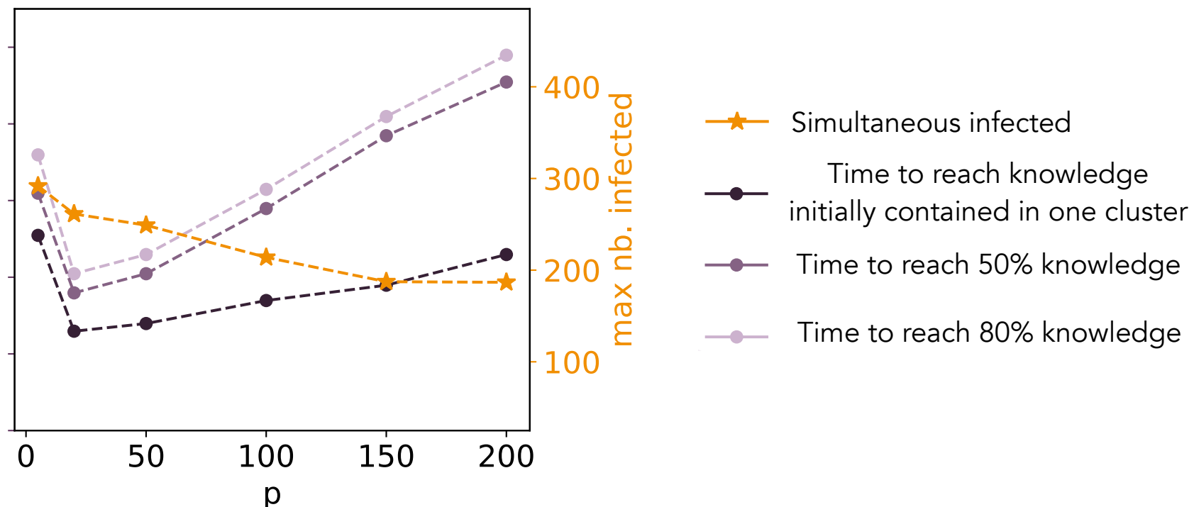
Bubbles
