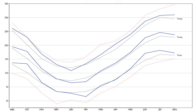
Température de l'air 2022 - 2023 (°C)
