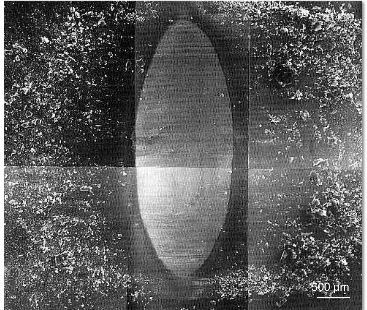
Production d'une grande quantité de débris (SSC-SSC, 40 N, 0,25 m/s, 500 m)
