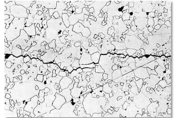
Propagation d'une fissure dans une alumine
