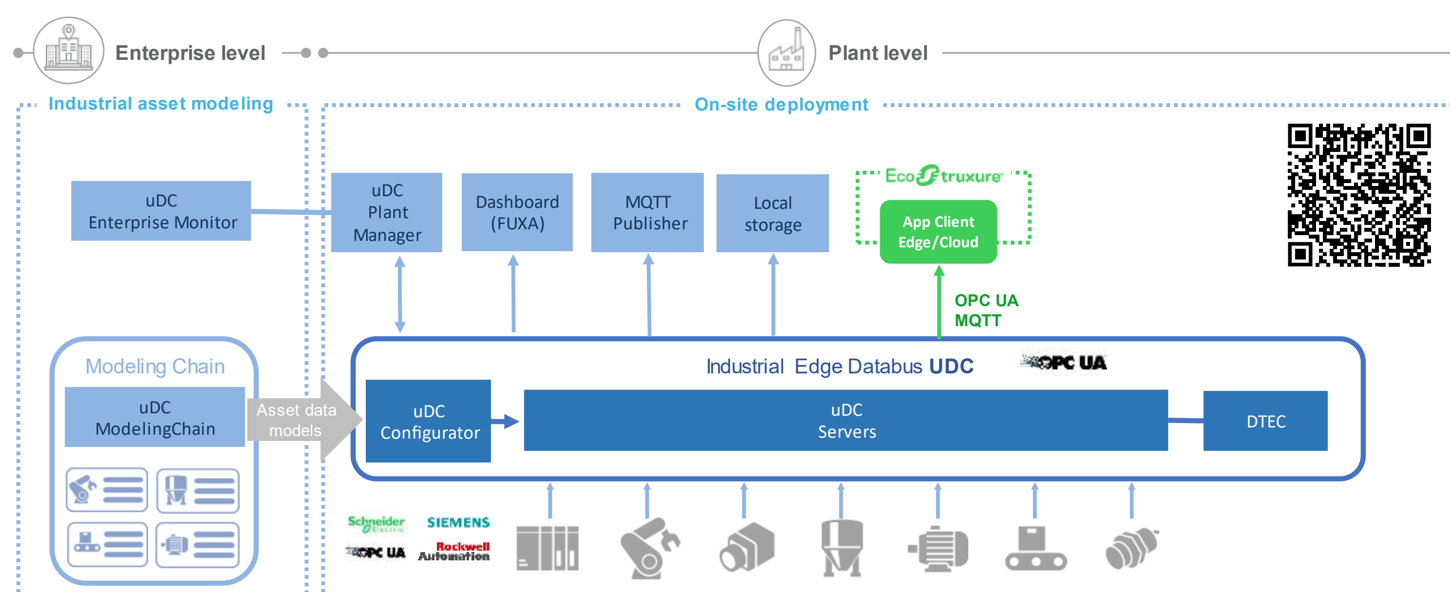
fig 3 : uDC Framework
