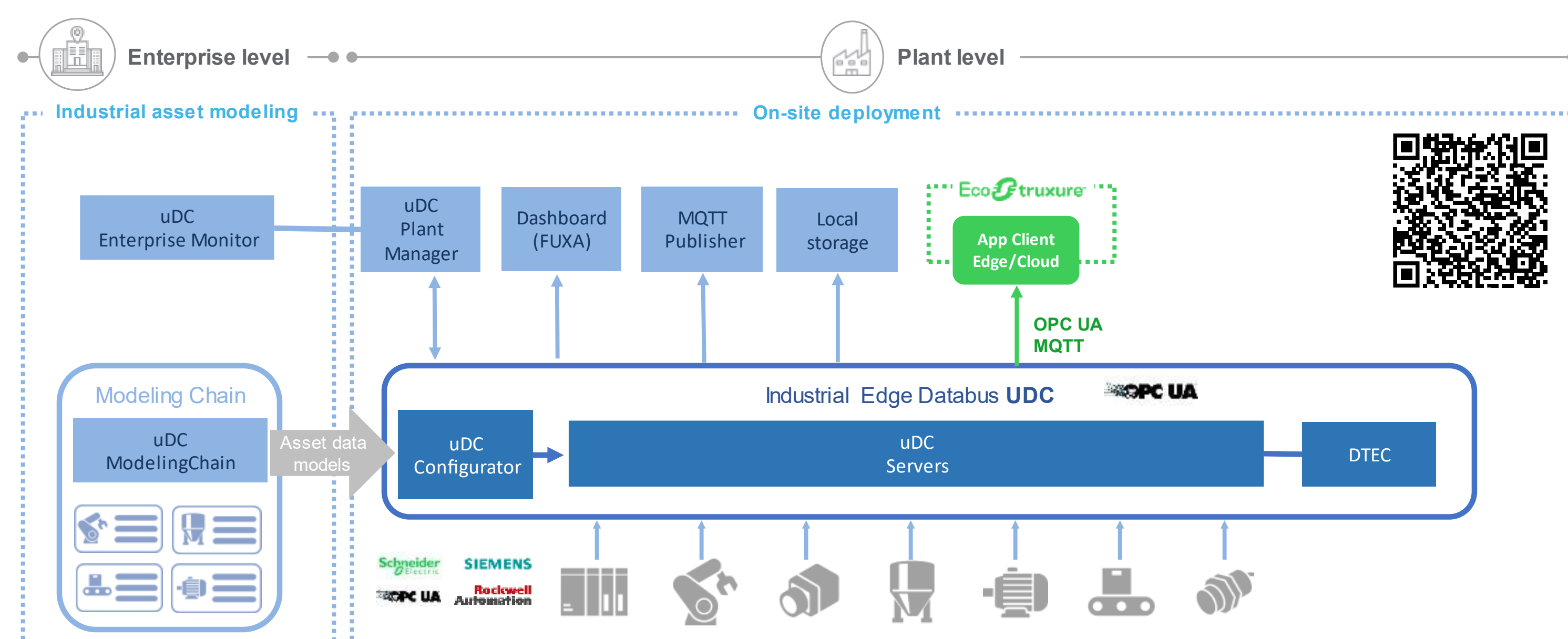
fig 3 : uDC Framework
