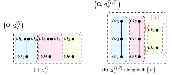
FIGURE 9 – \leq_{\varphi}^{\mathcal{T}_1} , le préordre partiel induit par la distance de Hamming aux modèles de \varphi de l'Exemple 7 au sein des cellules de Voronoï non ambiguë de la Figure 8 et \leq_{\varphi}^{\mathcal{T}_1, \mathcal{T}_2} , l'OLP obtenu après application du second tie-break avec \llbracket \alpha \rrbracket .
