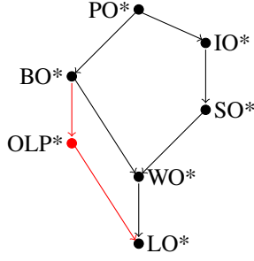
FIGURE 6 – Diagramme d’inclusions propres des parties asymétriques de structures ordonnées proposées dans [15]. PO = ordre partiel ; IO = ordre d’intervalles ; SO = semi-ordre ; BO = ordre bilinéaire ; OLP = ordre linéaire partitionné ; WO = ordre fort ; et LO = ordre linéaire. R* étant la partie asymétrique de la relation R.
