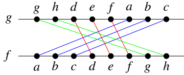
FIGURE 3 – Représentation graphique des fonctions f et g .
