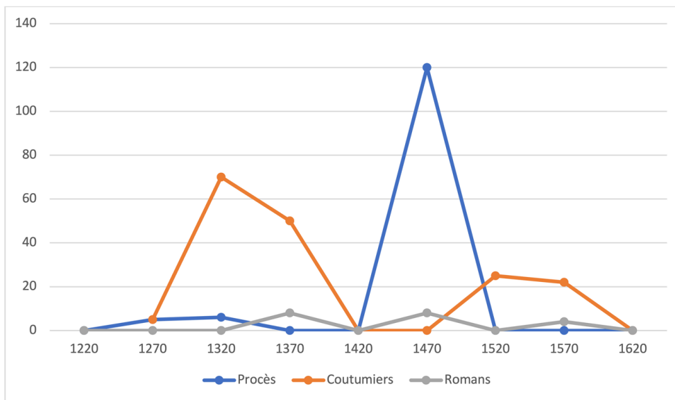
Graphique 2. Évolution des infinitifs antéposés dans les trois types de texte
