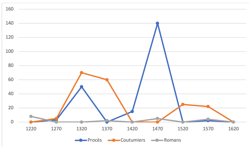
Graphique 1. Évolution des participes antéposés dans les trois types de texte
