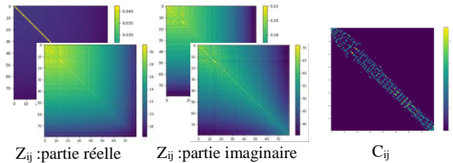
Fig.2. Matrices d'impédance magnétique et de capacité pour l'encoche B1
