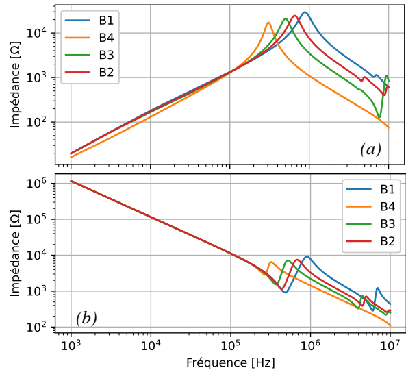
Fig.4. Impédance MD (a) et MC (b) obtenue pour les différentes configurations de bobinage
