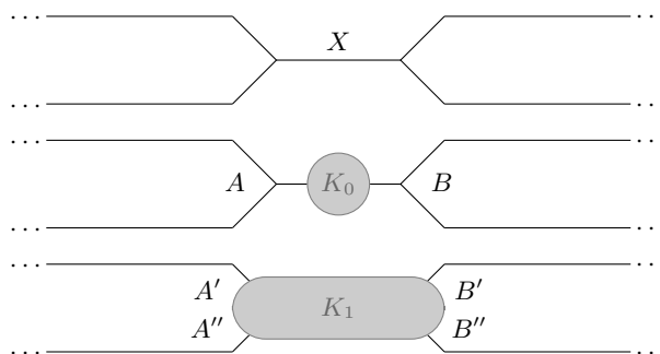
Fig. 8. K_0 \subseteq K_1 ; A', A'' \mapsto A ; B', B'' \mapsto B
