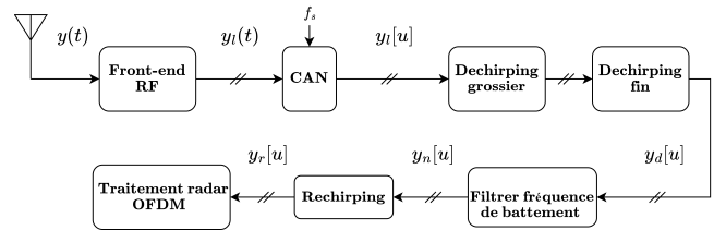
FIGURE 2 : Diagramme de suppression d'interférence.
