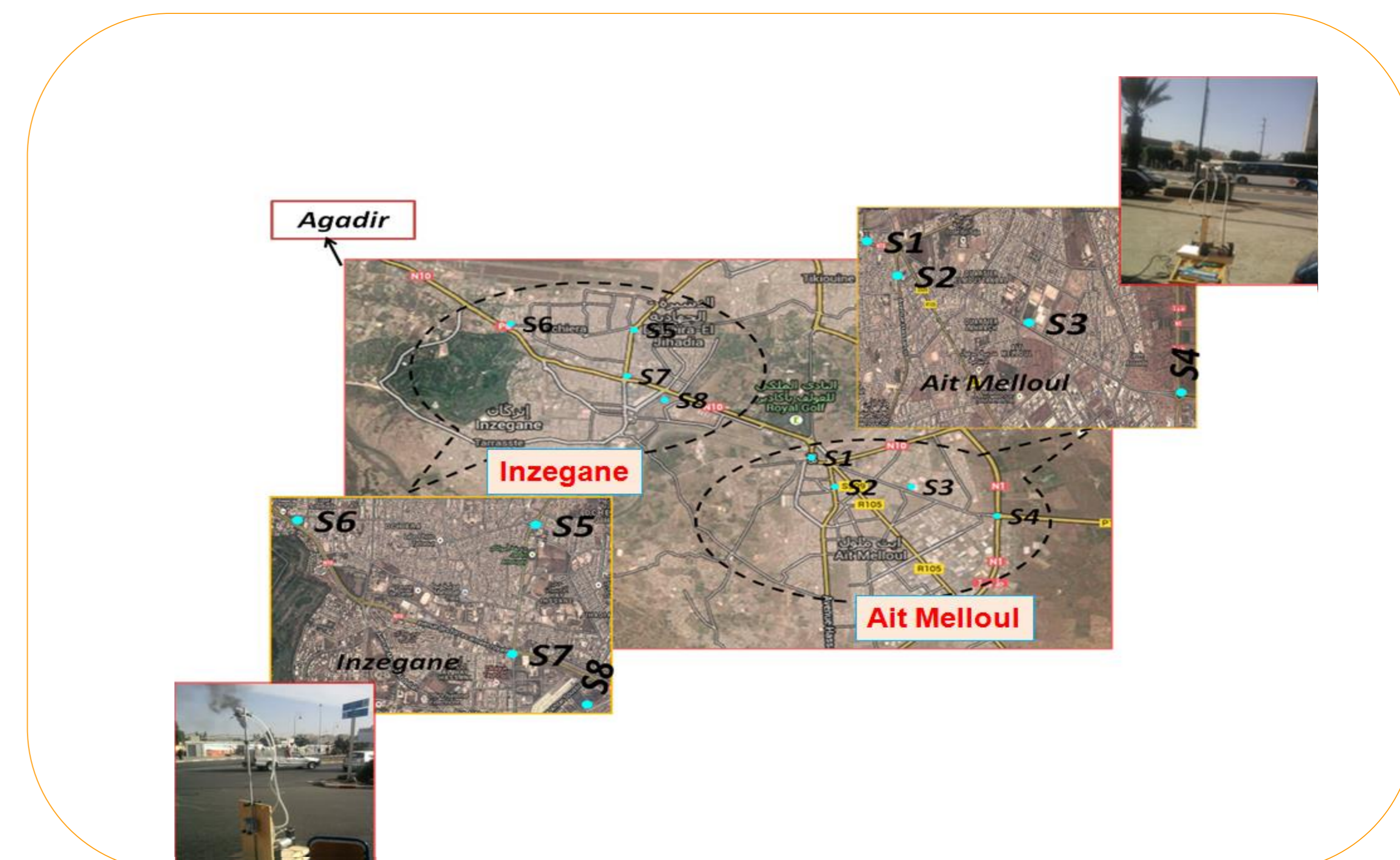
Fig. 1: Localisation des points de prélèvement sur la carte d'Inzegane Ait Melloul.
