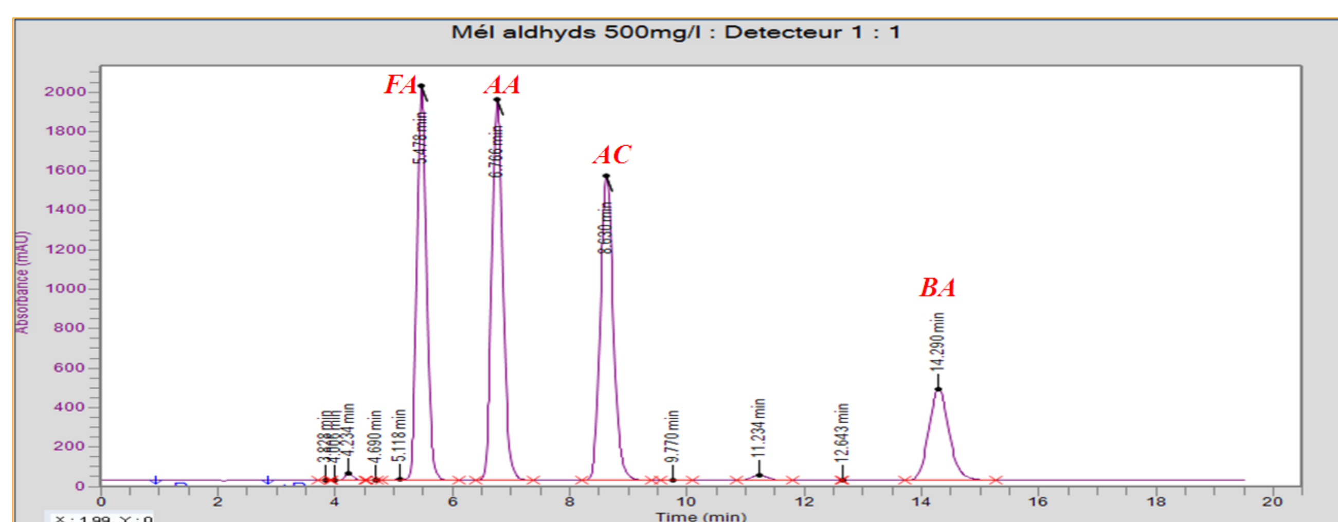
Fig. 2: Exemples des chromatogrammes des dérivés d'hydrazone et des BTX préparés et utilisés pour les courbes d'étalonnages.
