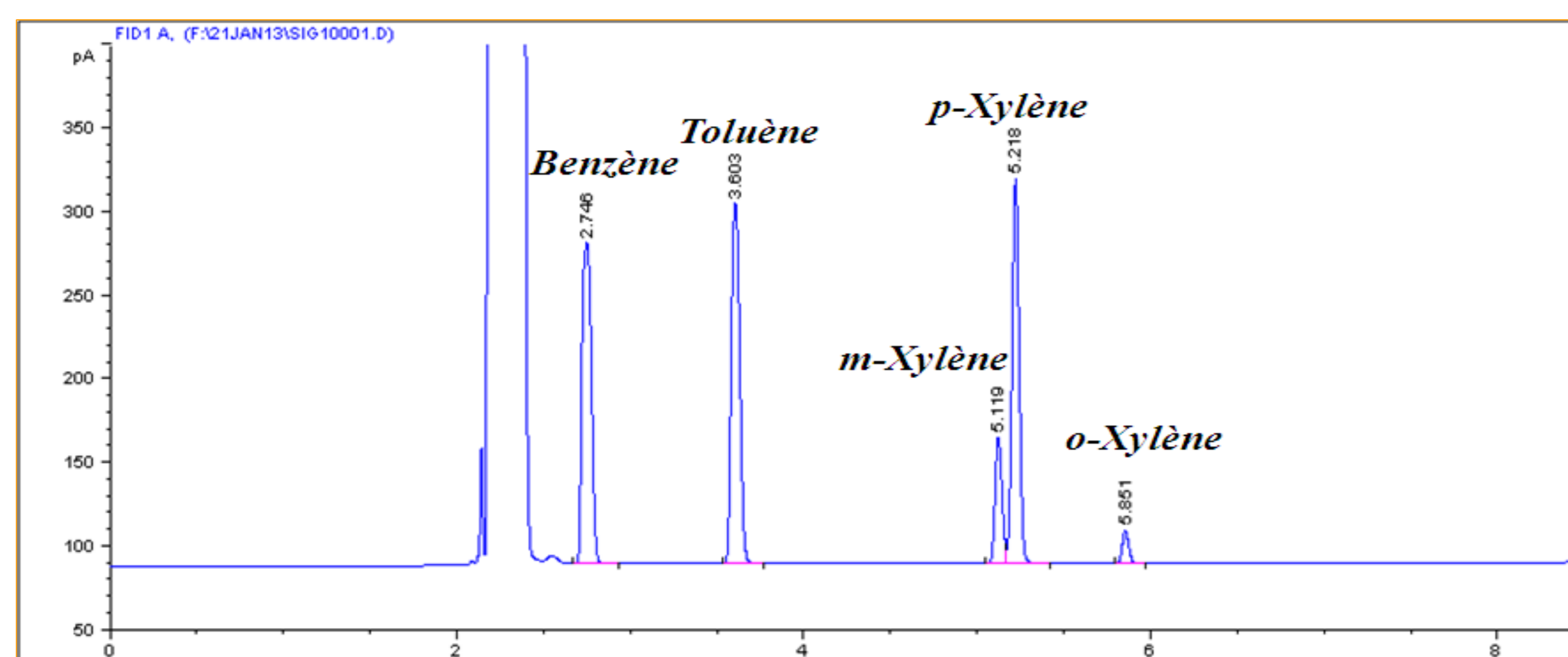
Fig. 3: Exemples des chromatogrammes des BTX préparés et utilisés pour les courbes d'étalonnages.
