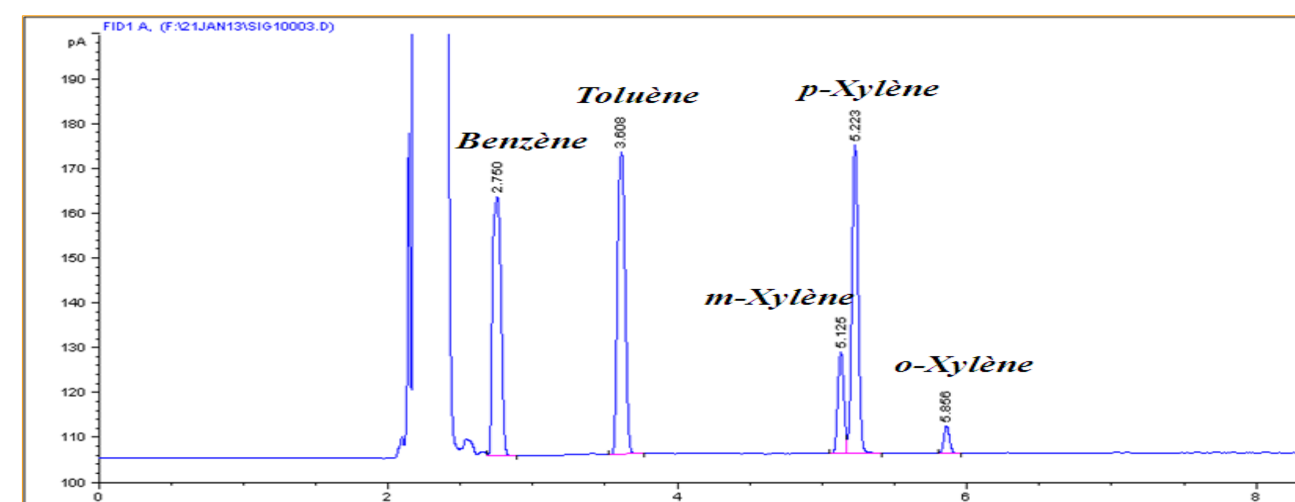
Fig. 4: Chromatogrammes des BTX pour un échantillon d'air prélevé dans le site n°9, le 22 novembre 2012, 14h15min -15h45min, T=16°C.
