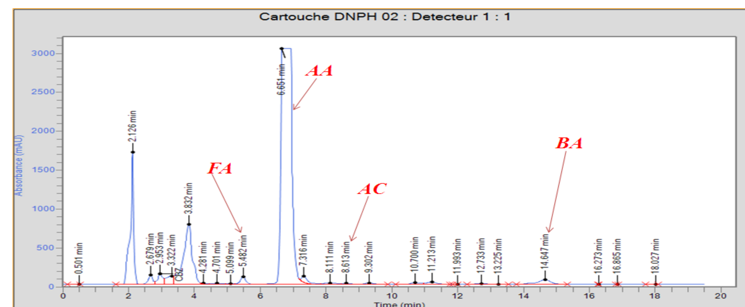
Fig. 5: Chromatogrammes des dérivés des hydrazone pour un échantillon d'air prélevés dans le site n° 6, le 23 novembre 2012, 9h17min à 12h17min, T= 20 ° C.
