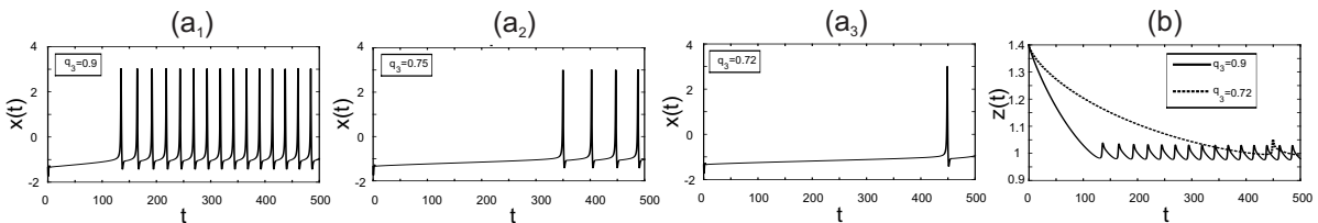
FIGURE 3. Contrôle du déclenchement et de l'activité électrique à l'aide de l'ordre fractionnaire q_3 du sous-système lent. Le potentiel transmembranaire x(t) produit 15 potentiels d'action pour q_3 = 0,9 (a 1 ), 4 potentiels d'action pour q_3 = 0,75 (a 2 ) et un potentiel d'action pour q_3 = 0,72 (a 3 ). La concentration en \text{Ca}^{2+} z(t) pour q_3 = 0,9 et q_3 = 0,72 est précisée à la sous-figure (b). Les autres paramètres sont a = \frac{1}{4} , \beta = 4 , \varepsilon = 0,0025 , u_\beta = -0,954 , \eta = 1 et q_1 = q_2 = 1 .
