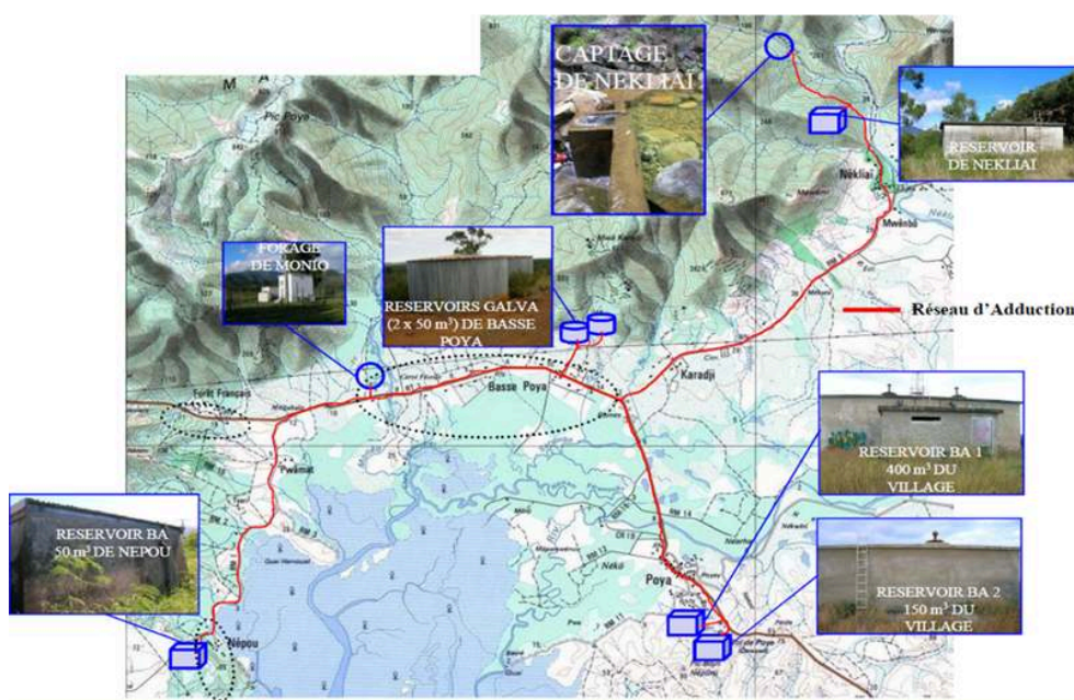
Figure 6. Rattachement du réseau de la tribu de Nékliaï au réseau communal de la commune de Poya
