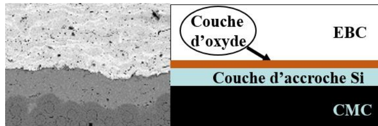
Fig. 1. Système CMC/EBC étudié
