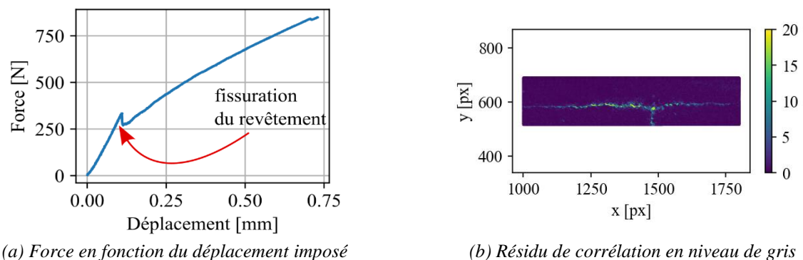
Fig. 3. Réponse macroscopique et champ de résidu mettant en évidence la présence de fissures dans le revêtement et à l’interface
