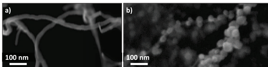
Figure 1 : Images FEG-SEM de MWCNTs (a) bruts et (b) décorés de nanoparticules de Cu
