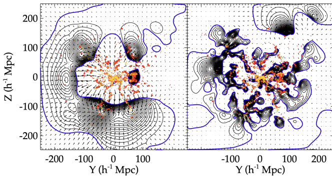
FIGURE 4 : Plan supergalactique YZ d'une reconstruction des champs de surdensité (contours) et de vitesse (flèche) de l'Univers local. La couleur bleue délimite les zones surdensités et celles sous-denses. Les points rouges sont les galaxies isolées du catalogue de redshift 2MRS [3] et les amas et groupes de galaxies de [6]. Les points jaunes correspondent aux galaxies des catalogues biaisé (gauche) et corrigé (droite).
