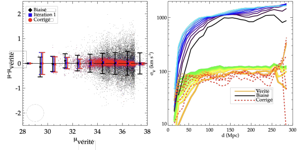
FIGURE 2 : Gauche : Différence entre modules de distance vrais et i) biaisés (losanges noirs), ii) après une itération du recuit simulé (carrés bleus), iii) corrigés (cercles rouges) en fonction des vrais. Droite : Variance des vitesses aux petites échelles dans des volumes, V (une ligne par élongation) pour un catalogue sans erreur (vérité, lignes continues aux couleurs chaudes), avec des erreurs (biaisé, lignes continues aux couleurs froides), après application de l'algorithme (corrigé, lignes pointillées). La variance est celle des vitesses des galaxies appartenant à un même volume V , d'élongation proportionnelle à une incertitude sur le module de distance de valeur 0,2 (orange, rouge, noir) à 1,8 (vert, orange, bleu) mag.
