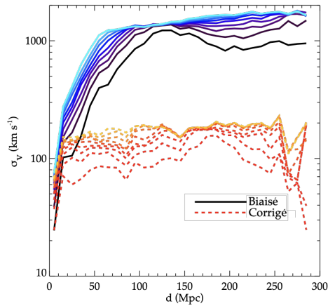
FIGURE 3 : Comme Fig. 2 droite mais pour le catalogue observationnel.
