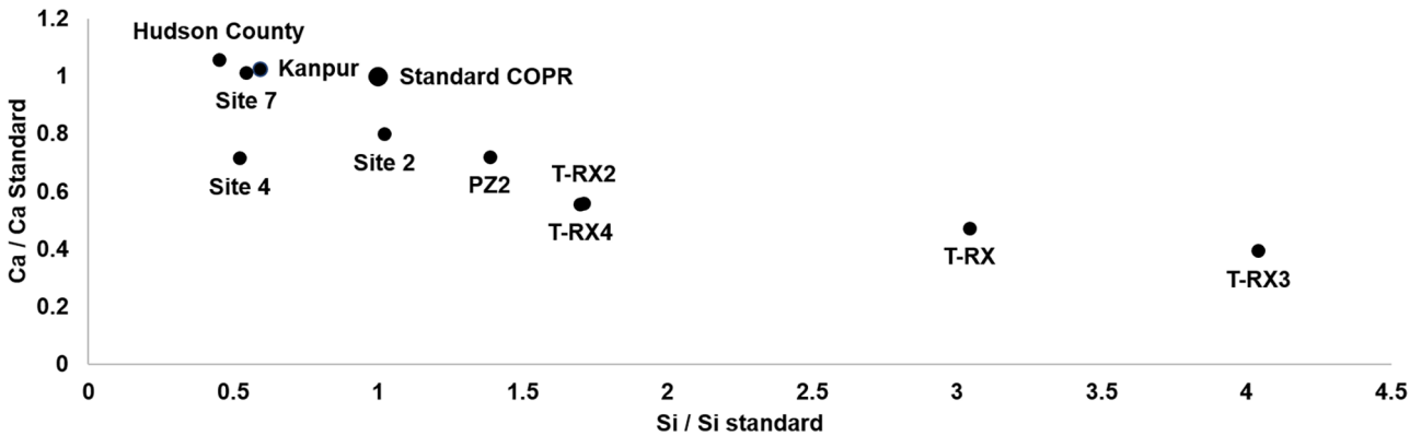
Fig. 1. Comparison of “our” COPR and COPR from sites published in the literature with “standard COPR”. All data used are given in Table 1 . Fig. 1. Comparaison des charrées de chrome de cette étude et de charrées d’autres études avec les « charrées de chrome standard ». Les données proviennent du tableau 1 .
