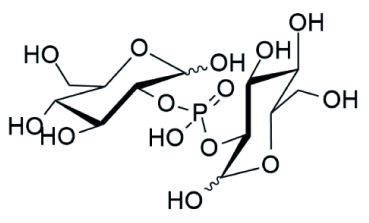
AgroD-like2
