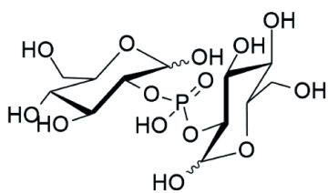
AgroD-like2
