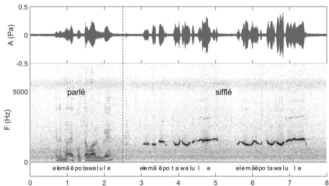
Figure 4 : Phrase wayāpi / elemāē po tawalu le /, parlée puis sifflée deux fois. Forme d'onde (en haut) et spectrogramme (en bas) montrant une même phrase wayāpi parlée (de 0 à 2.5 sec.) puis sifflée deux fois (2.5 à 5 sec., puis de 5.3 à 7.5 sec.). / elemāē po tawalu le / signifiant "As-tu vu une tortue d'eau ?" 8 , où / tawalu / est la tortue d'eau. On observe ici les mêmes caractéristiques linguistiques que pour la Figure 3, avec cette fois-ci une répétition de la phrase sifflée. La répétition est plus précise, en particulier dans les premières syllabes. On observe aussi un allongement et une plus forte intensité de la dernière syllabe / le /, lui conférant un effet emphatique. Cet enregistrement a été réalisé sur une pirogue située sur la rivière, non loin de la berge, et l'on observe que les répétitions sifflées se placent en fréquence juste au-dessus des fréquences basses du bruit de fond ambiant de plus forte intensité (zone sombre dans la partie basse de la figure) et bien au-dessous de la bande stationnaire des insectes située un peu au-dessus de 5000 Hz. Par contre, la version parlée, elle, est plus masquée par le bruit ambiant.
