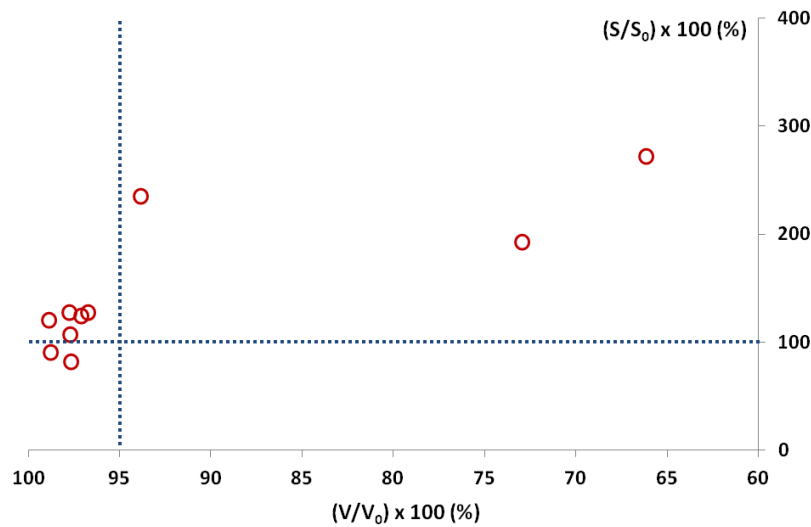
Figure 10 : Variation de la sorptivité ( S/S_0 ) en fonction de la variation de la vitesse sonique ( V/V_0 ) mesurée sur les éprouvettes témoins 11 x 22 cm.
