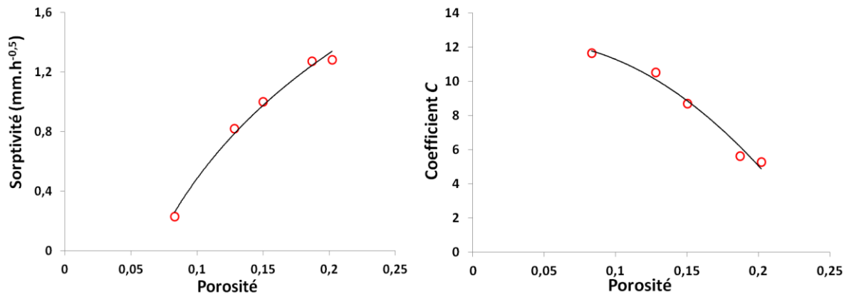
Figure 4 : Evolution de la sorptivité (à gauche) et du coefficient C (à droite) en fonction de la porosité des bétons.
