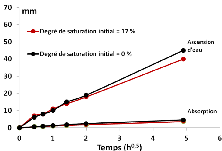
Figure 6 : Absorption et ascension de l'eau pour un degré de saturation initial de 0 et 17%.
