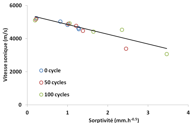
Figure 9 : Evolution de la vitesse sonique en fonction de la sorptivité.
