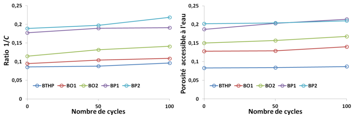
Figure 11 : Evolution du ratio 1/C (à gauche) et de la porosité accessible à l'eau (à droite) en fonction des cycles gel-dégel.
