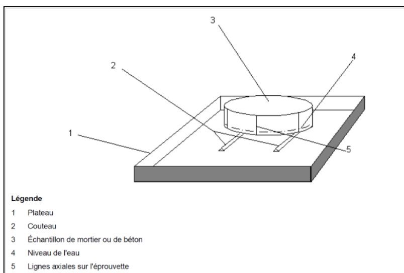
Figure 1 : Illustration de l'essai d'absorption capillaire (extraite de la norme NF EN 13057).
