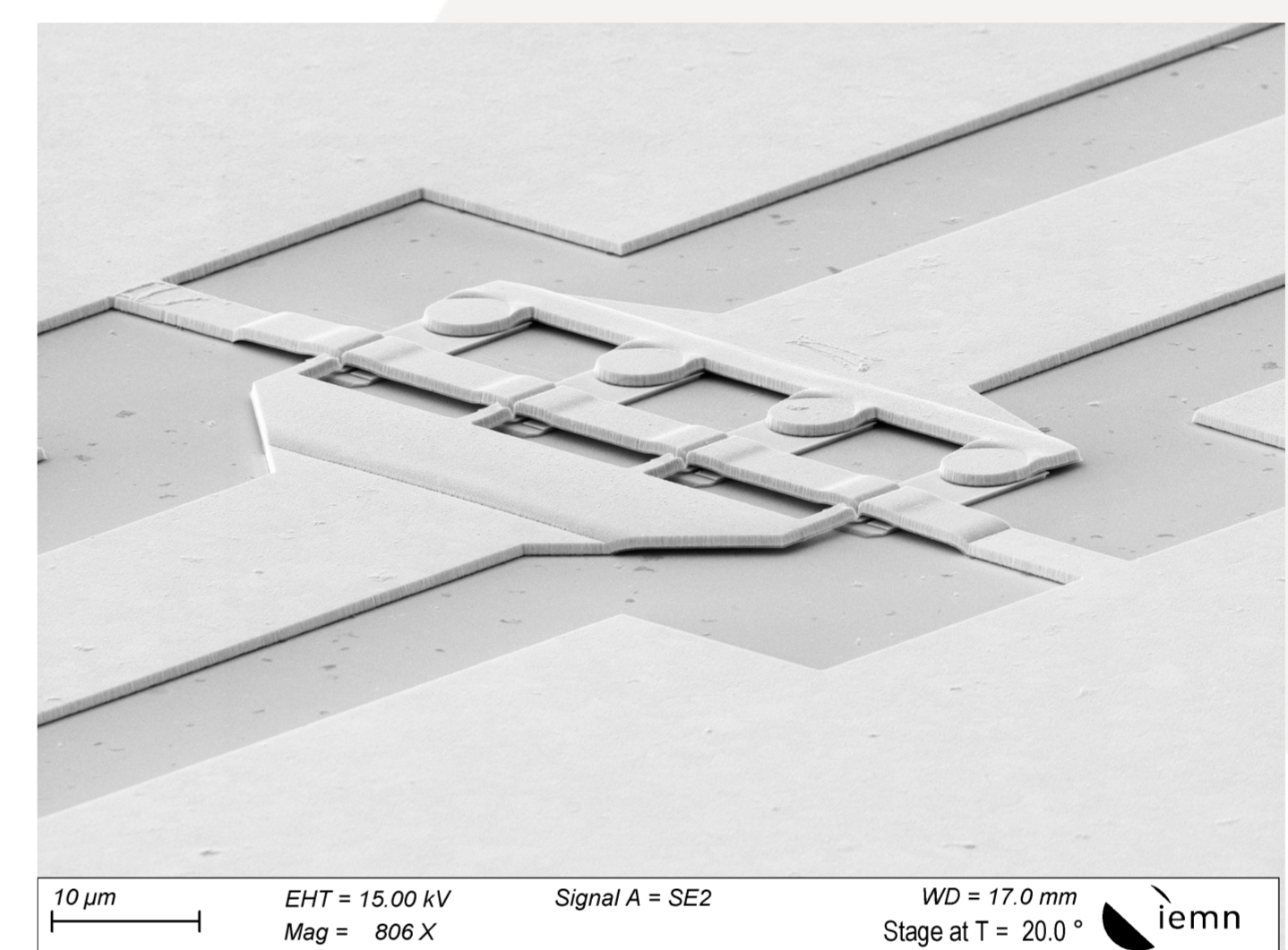
Process III-V sur InP & Si
