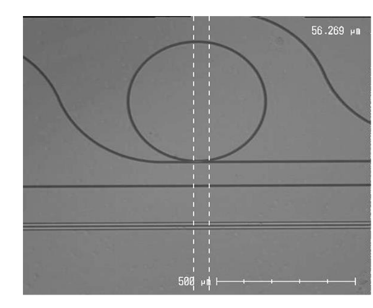
INL, Leti, Résonateur SiGe
