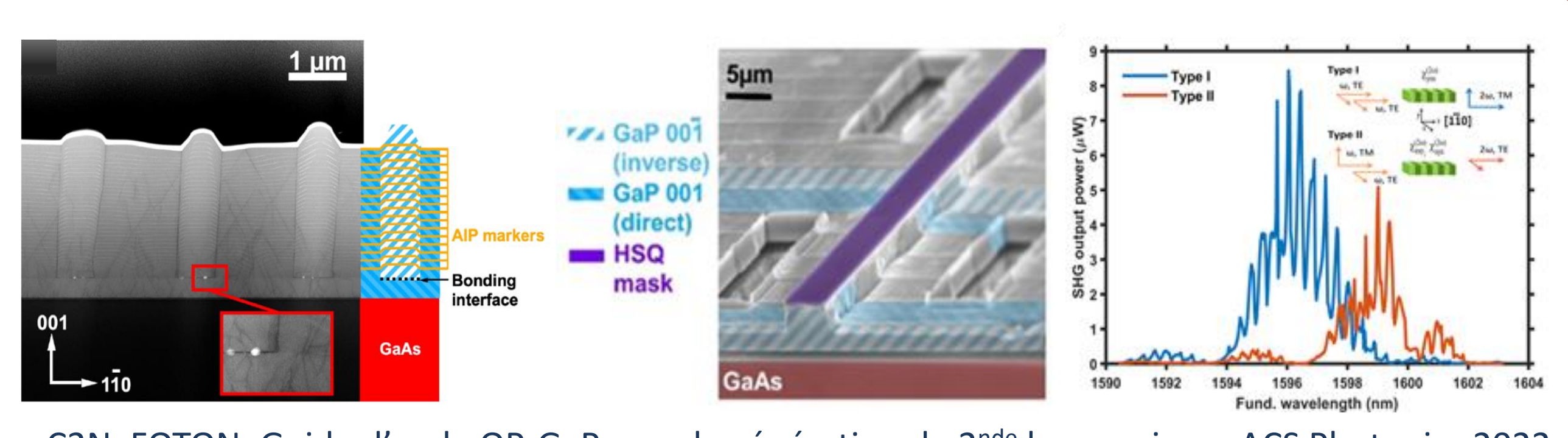
C2N, FOTON, Guide d'onde OP-GaP pour la génération de 2 nd e harmonique, ACS Photonics 2022
