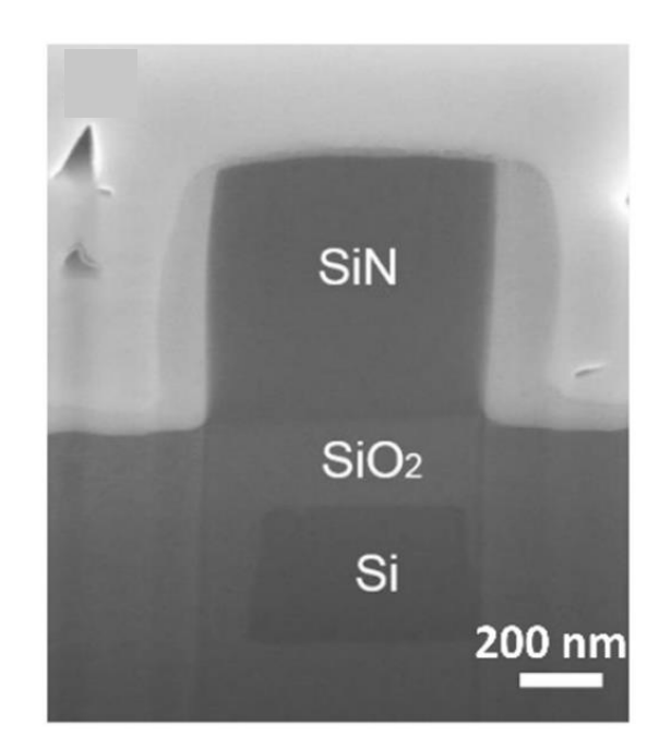
Leti, stratégies de co-intégration Appl. Science 2019
