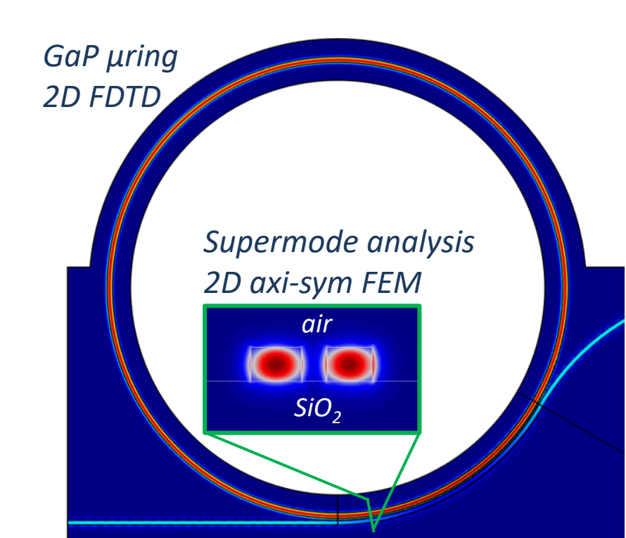
FOTON, design de coupleurs pour résonateurs GaP
