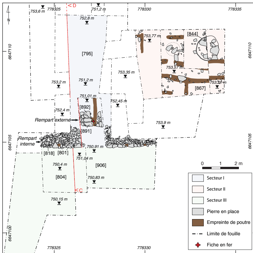
2. BibRACTE, Mont-Beuvray. Les Grandes Portes. Sondage dans le rempart interne. Orthophotographie de fin de fouille et plan général des secteurs (DAO Cl. Filet; orthophotographie BibRACTE/A. Meunier).
