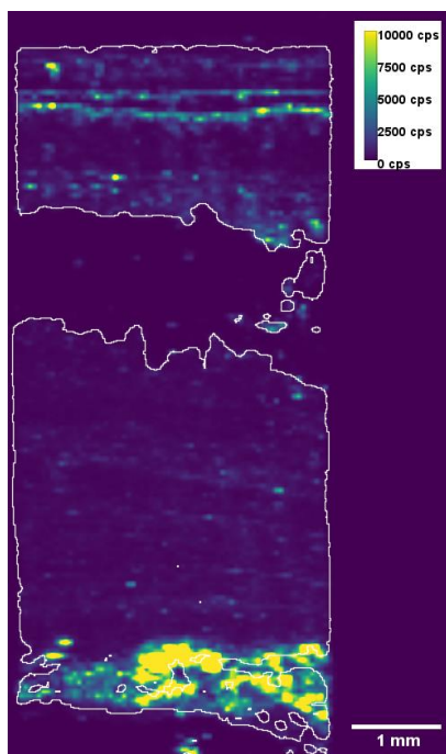
(d) ^{232}\text{Th}
