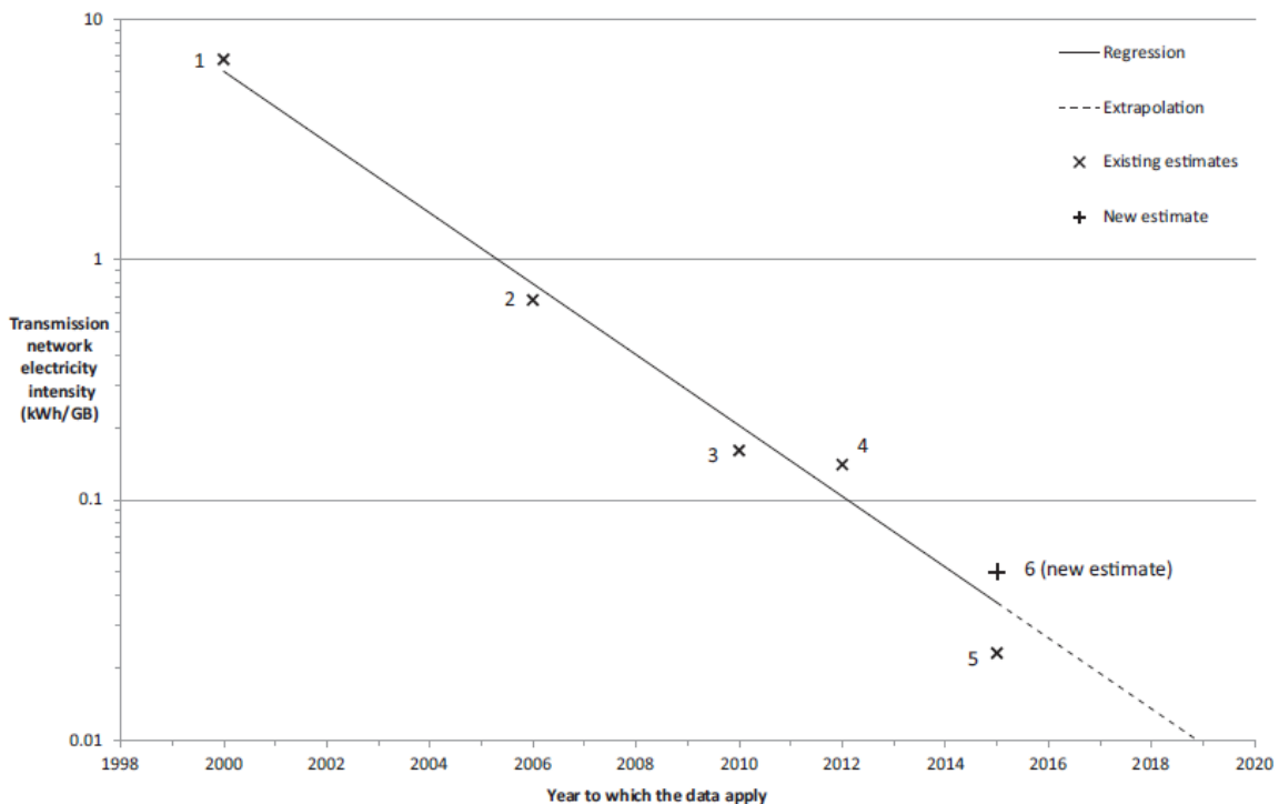
Figure 11 - Consommation d'énergie par GB transporté sur les réseaux de transmission (13)
