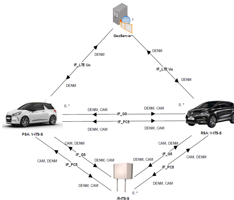
Figure 15 - schéma de communication de la fonction étudiée
