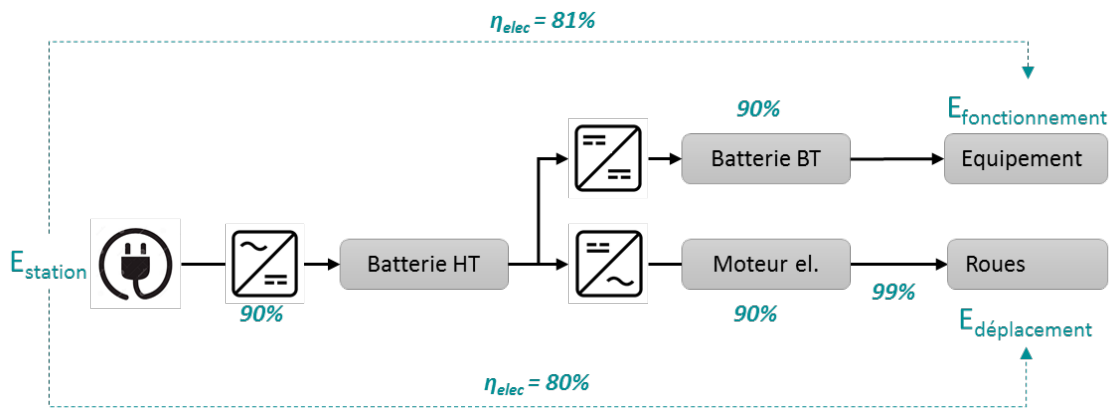
Figure 24 - rendements énergétiques véhicule électrique
