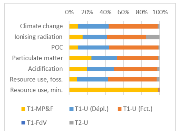
Figure 19 - répartition des impacts environnementaux de la FC sur un véhicule diesel
