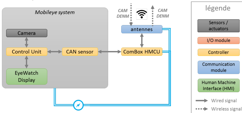
Figure 16 - schéma fonctionnel équipements véhicule (tiers 1 IoV)
