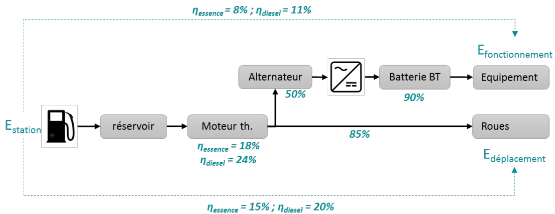
Figure 25 - rendements énergétiques véhicules thermiques
