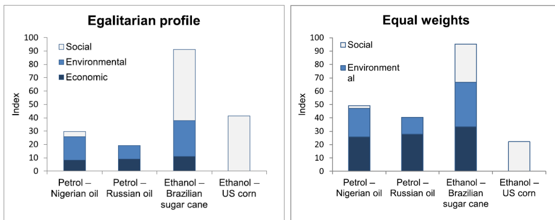
Figure 14 – résultats de LCSA de carburants (28) avec et sans pondération entre les 3 aspects de la soutenabilité
