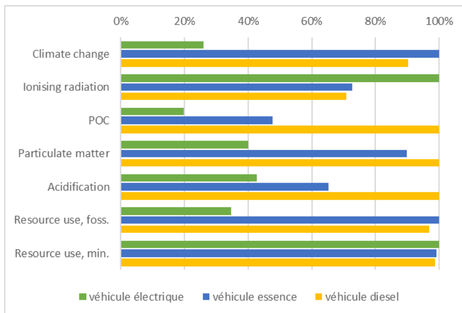
Figure 20 - comparaison des impacts de la fonction connectée évaluée par motorisation véhicule
