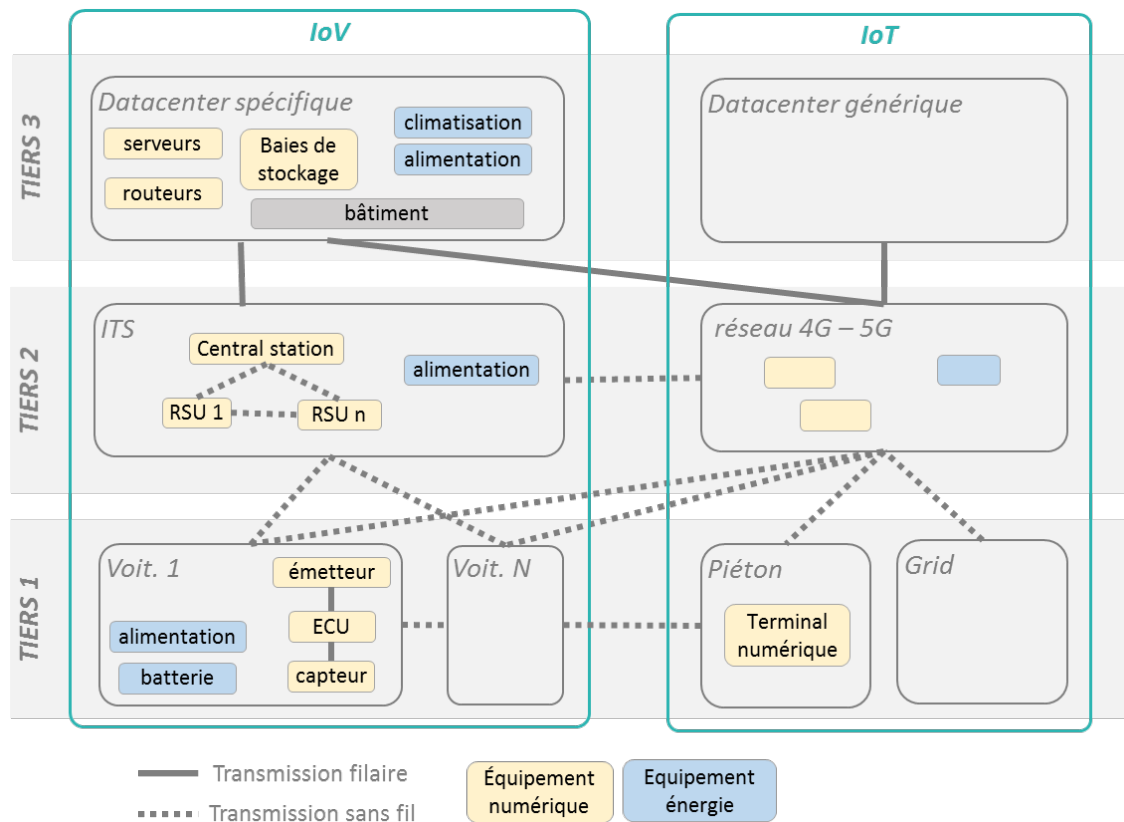
Figure 9 - périmètre physique de la fonction connectée
