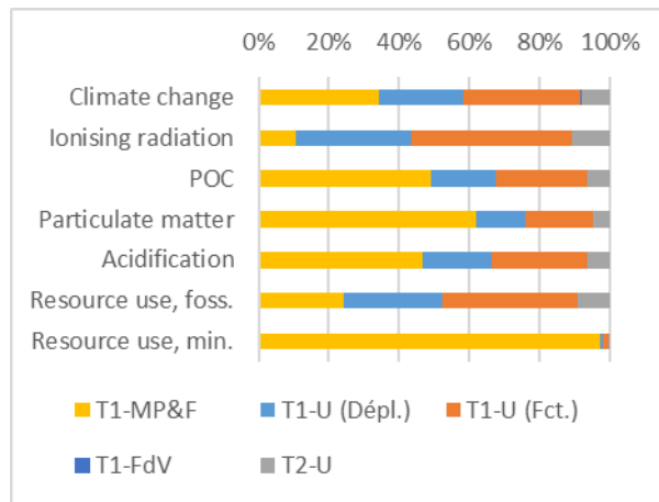
Figure 17 - répartition des impacts environnementaux de la FC sur un véhicule électrique
