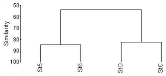
b) Abundance
