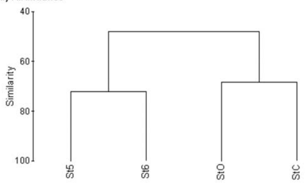
b) Abundance
