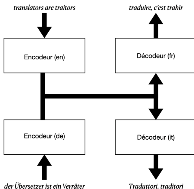
Figure 3. Une illustration de l'architecture encodeur-décodeur pour un système multisource-multicible, comprenant deux encodeurs et deux décodeurs. Ce système unique produit des traductions automatiques pour 4 couples de langues
